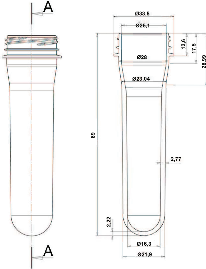
A-A View/Görünüm
